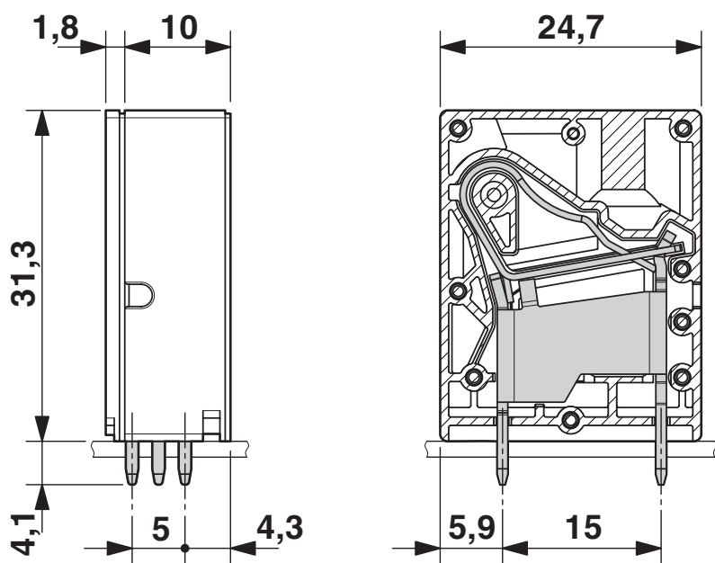
尺寸图
