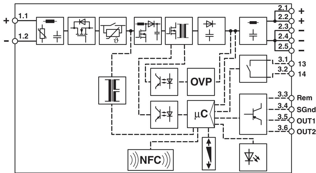
结构框图
