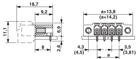
外形寸法
