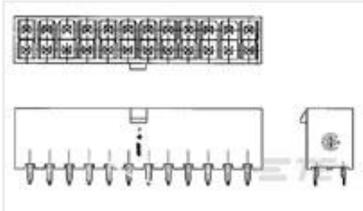
TE Part #1586768-2 2P VERT HDR VAL-U-LOK GW
