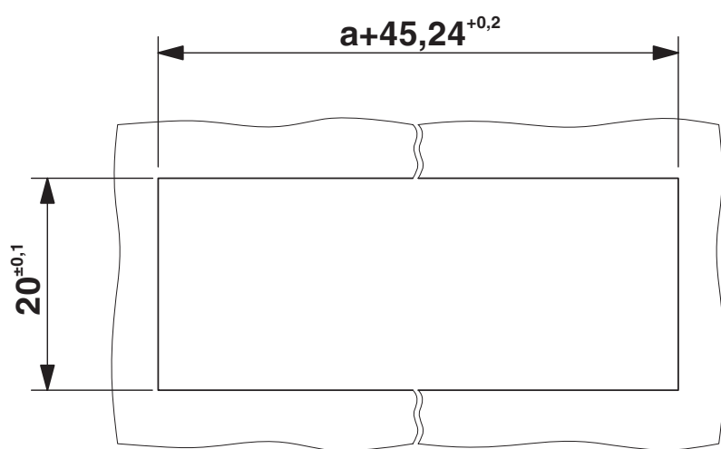
尺寸图
