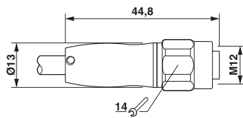
外形寸法
