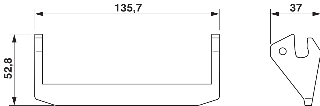
尺寸图
