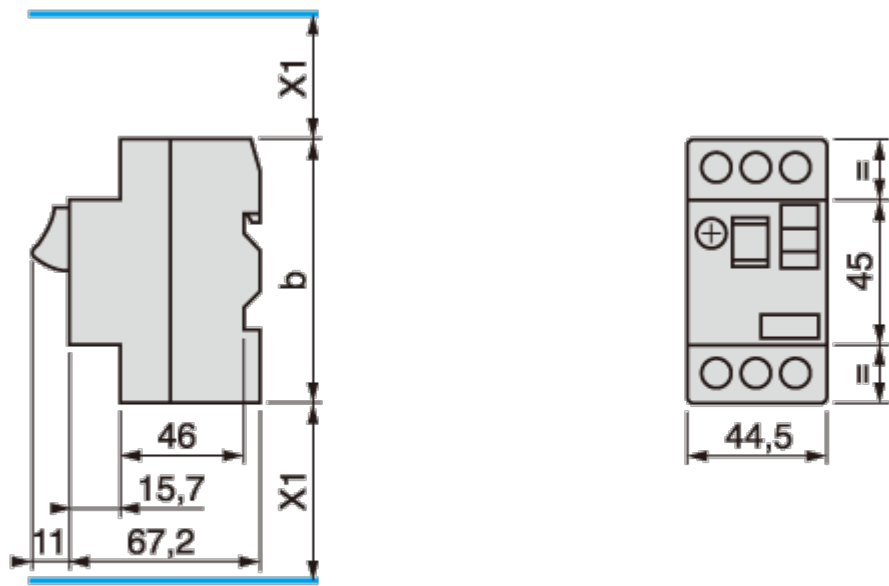
GV2ME
