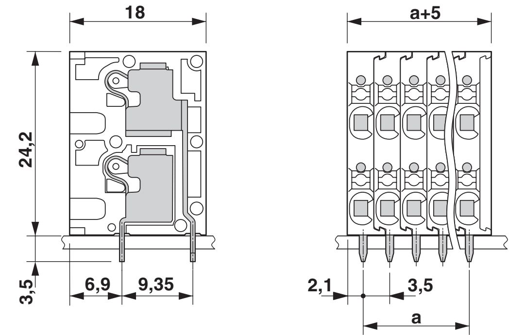
尺寸图
