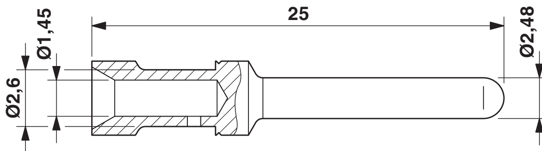
尺寸图
