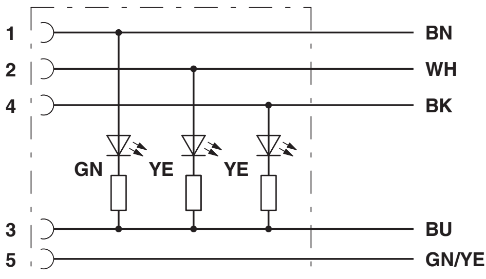
电路图
