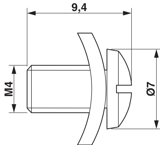
尺寸图
