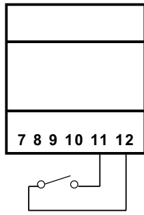
Digital_Input
