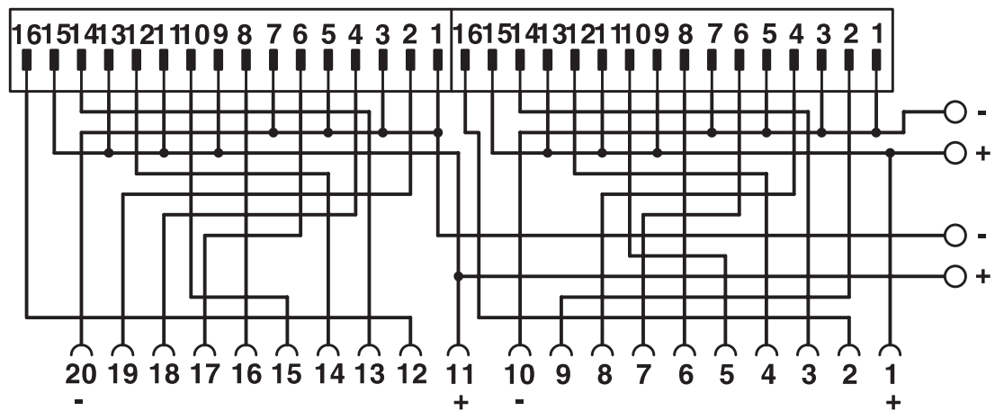
电路图
