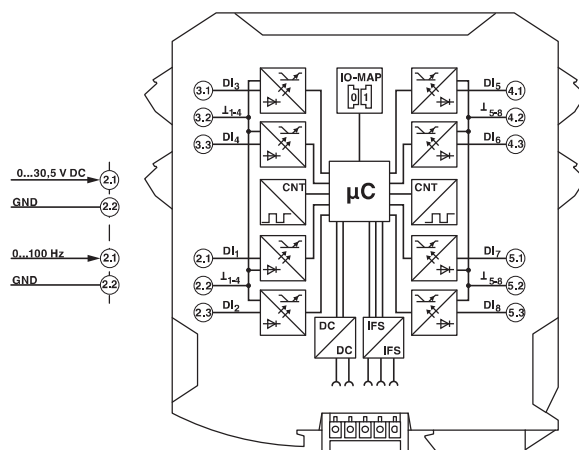
电路图
