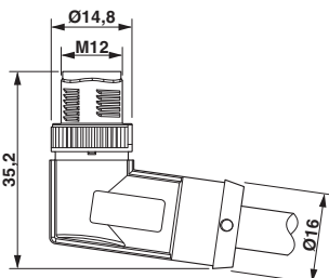
外形寸法
