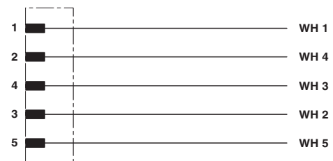
回路図
