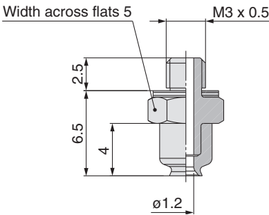
ZP2-T04AU□-A3
