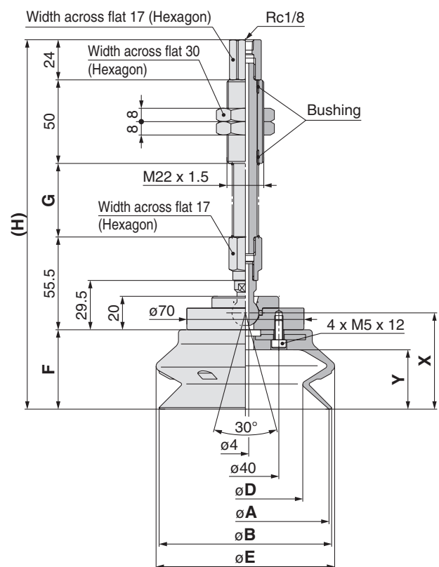
Dimensions
