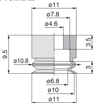
ZP2-B10MB
