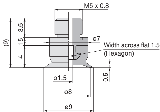
ZP2-T08EU□-H5
