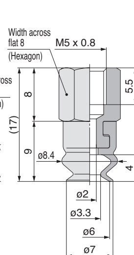
ZP2-TB06MB□-B5
