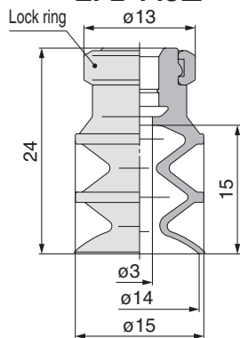
ZP2-14J
