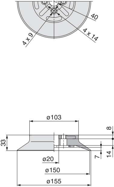
ZP2-150HT □
