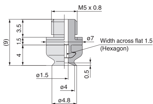
ZP2-TB04EU□-H5
