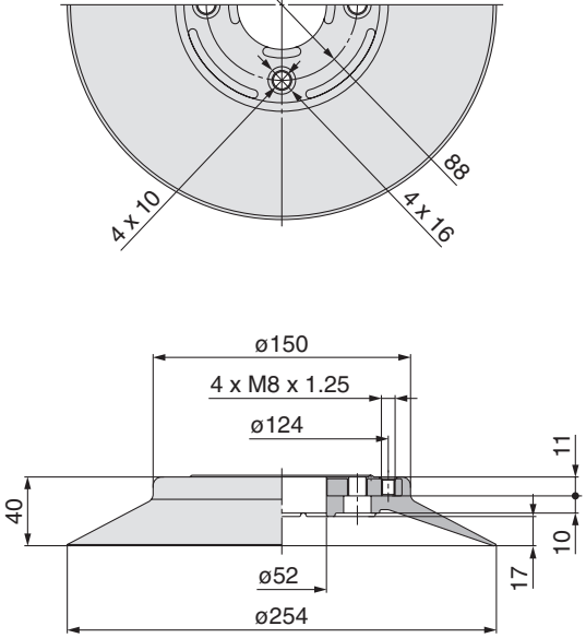
ZP2-250HT □
