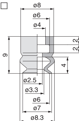
ZP2-B08MB
