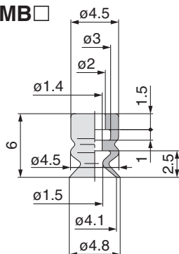
ZP2-B06MB
