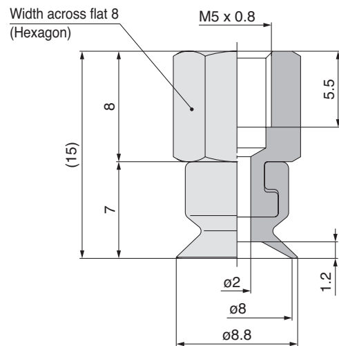
ZP2-TB08MU□-B5
