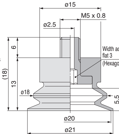
ZP2-TB20MB□-H5
