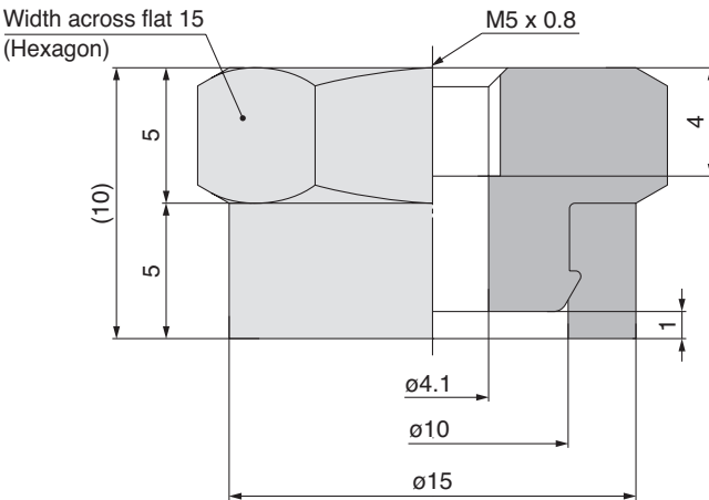
ZP2-T15S□GE-B5
