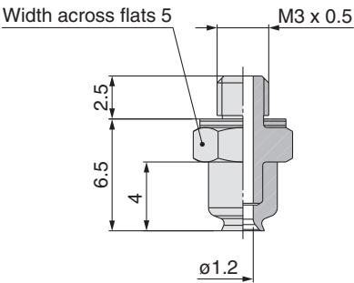
ZP2-T02AU□-A3
