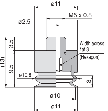
ZP2-TB10MB□-H5
