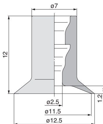
ZP2-11UT□
