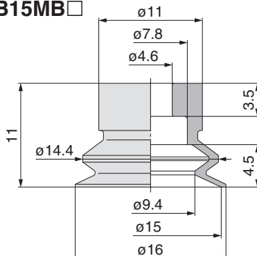
ZP2-B15MB
