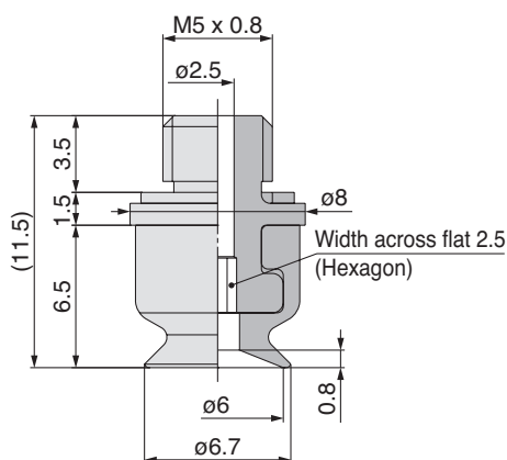
ZP2-TB06MU□-H5
