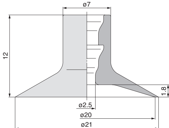
ZP2-20UT□
