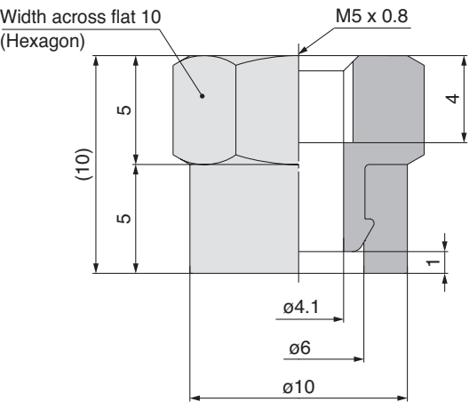
ZP2-T10S□GE-B5
