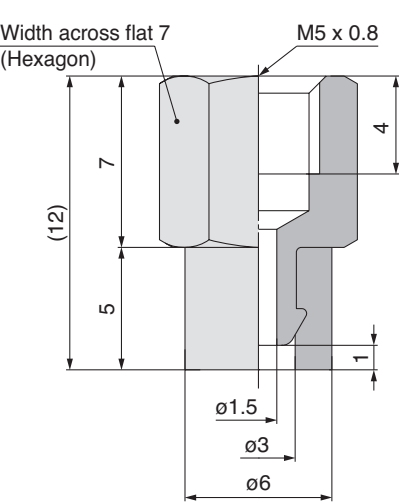
ZP2-T06S□GE-B5
