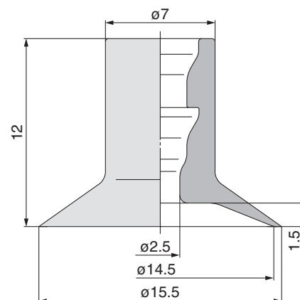
ZP2-14UT□
