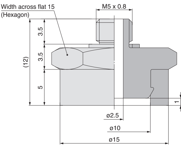
ZP2-T15S□GE-A5
