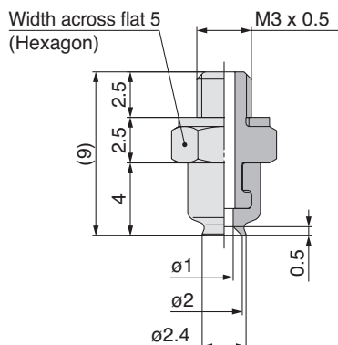
ZP2-TB02MU□-A3
