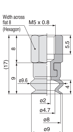
ZP2-TB08MB□-B5
