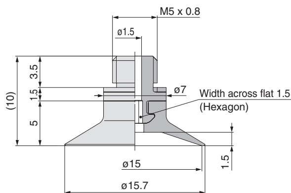
ZP2-T15EU□-H5
