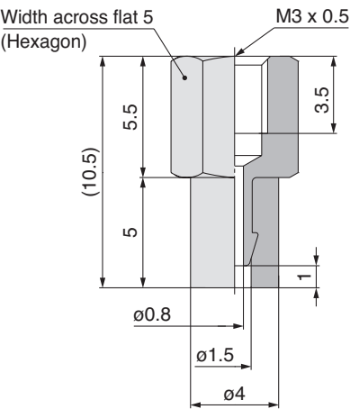
ZP2-T04S□GE-B3
