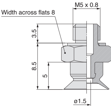
ZP2-TB08AU□-A5
