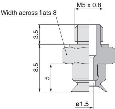
ZP2-T06AU□-A5
