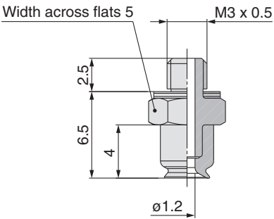
ZP2-T03AU□-A3
