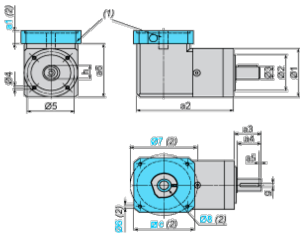
带伺服电机改装套件 的尺寸
