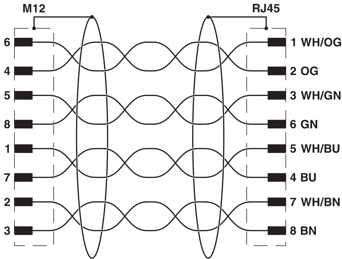
电路图
