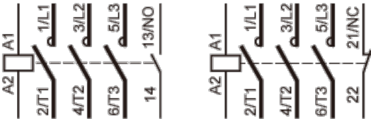
1NO+1NC(LANN11)
