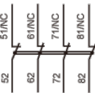
4NC(LANN04)
