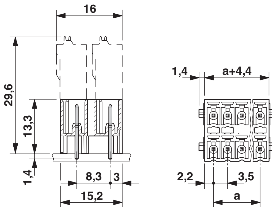
尺寸图
