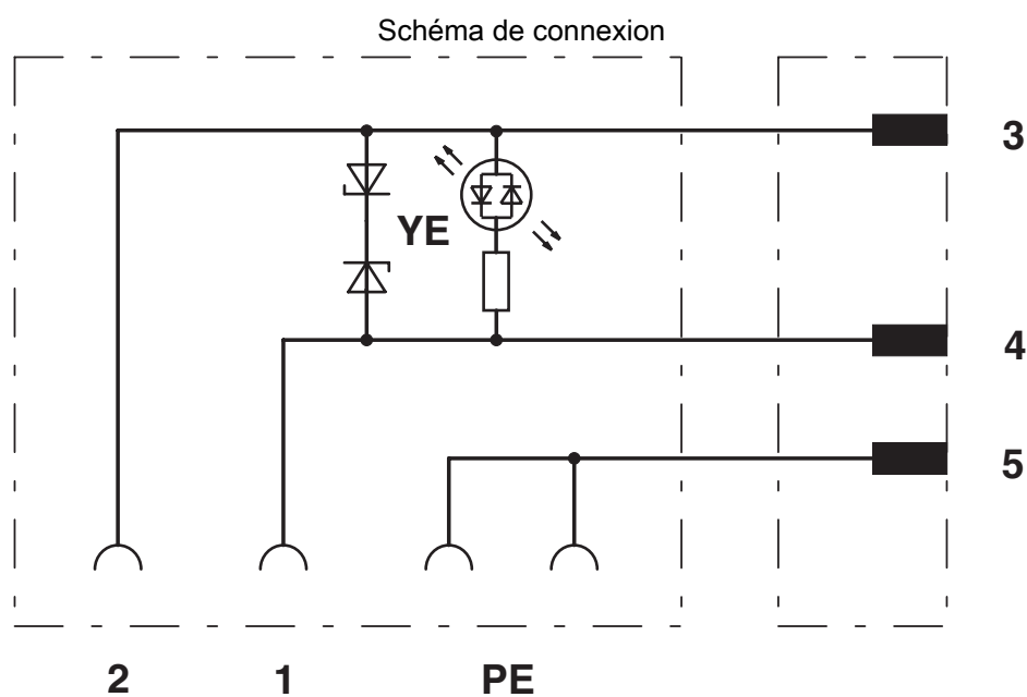
Connecteur pour électrovanne, type A
