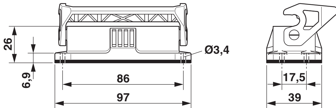
Maßzeichnung
