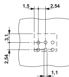
Bohrplan
