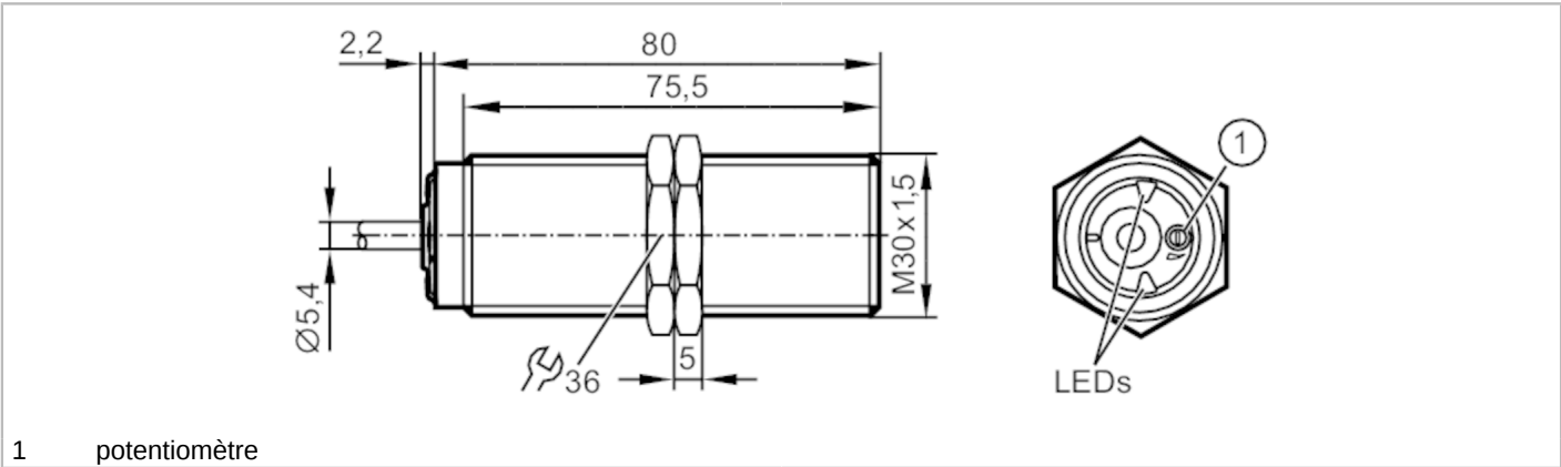
1 potentiomètre
