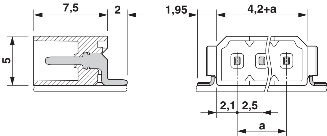
尺寸图
