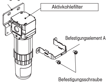
Befestigungselement B
