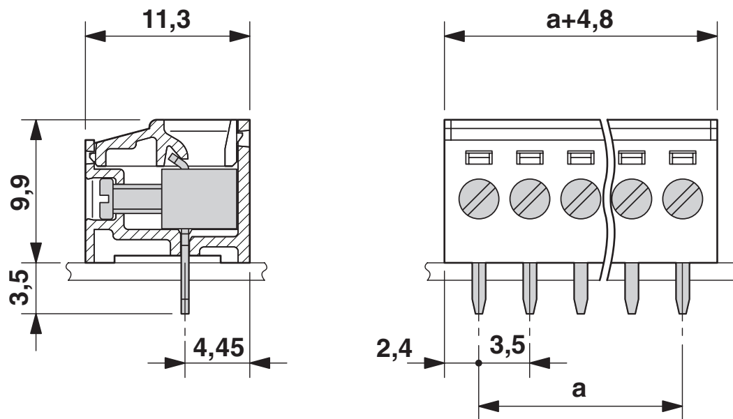
尺寸图
