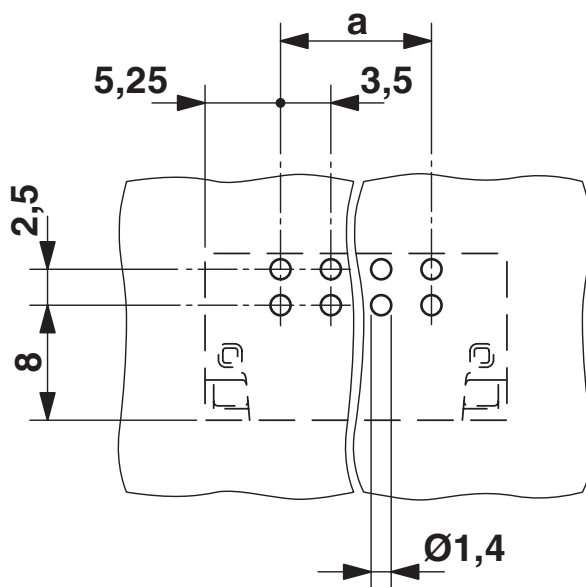
穴あけ加工図/ハンダパッドの形状
