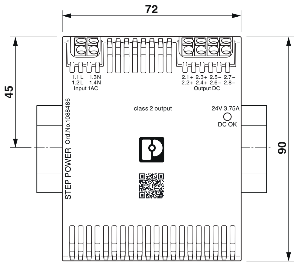
尺寸图
