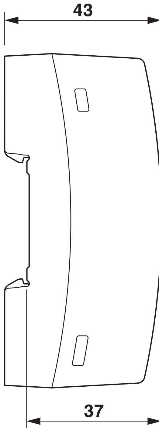
尺寸图
