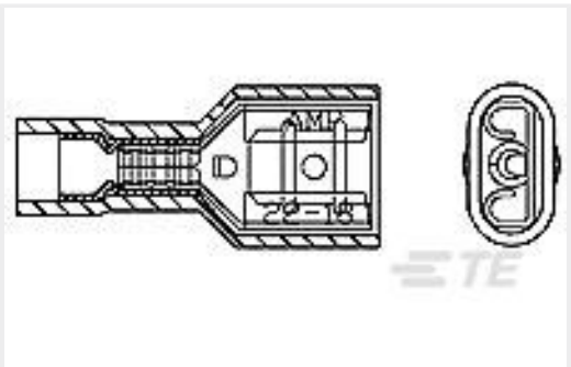
TE Part #735278 EPEZT * STECKHUELSE ISOLIERT 6,3 X 1,0 *
