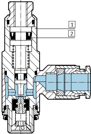
Valvola unidirezionale, pilotata
