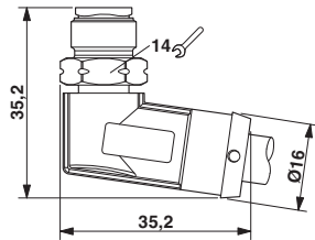
外形寸法
