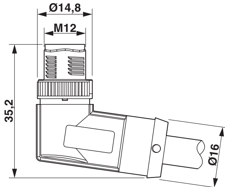
尺寸图
