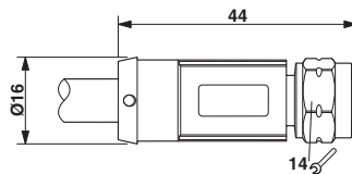
外形寸法
