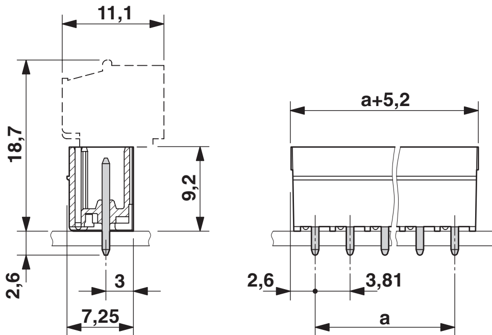
尺寸图
