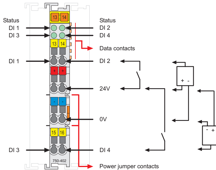
Fig. 2.1.1-1: 4- Channel Digital Input Module 750-402
