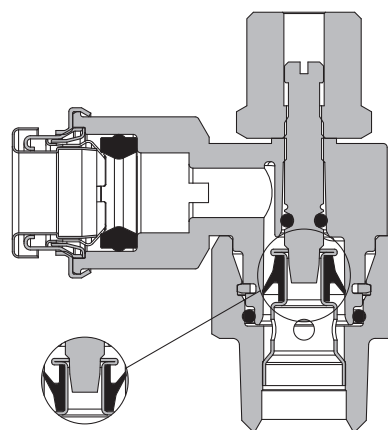
Réglage admission
