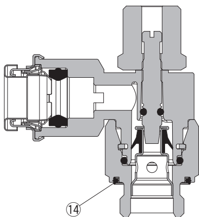
Réglage échappement
