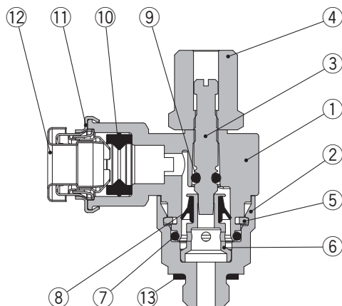
Réglage échappement
