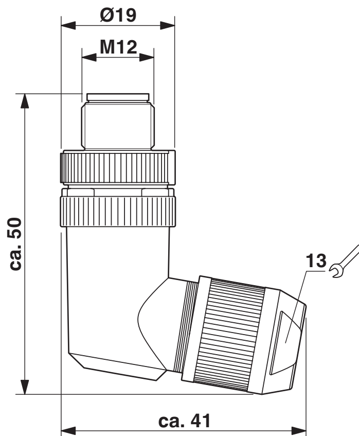
尺寸图
