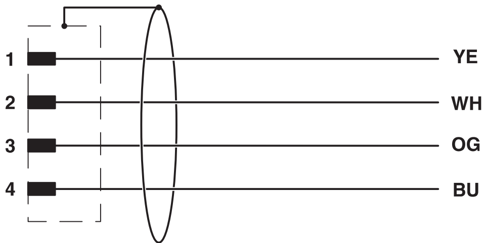
电路图
