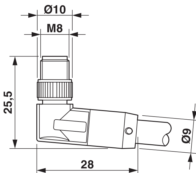
尺寸图
