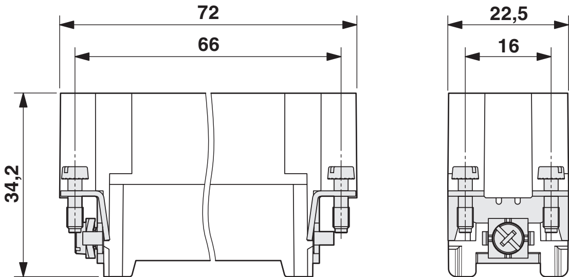
尺寸图
