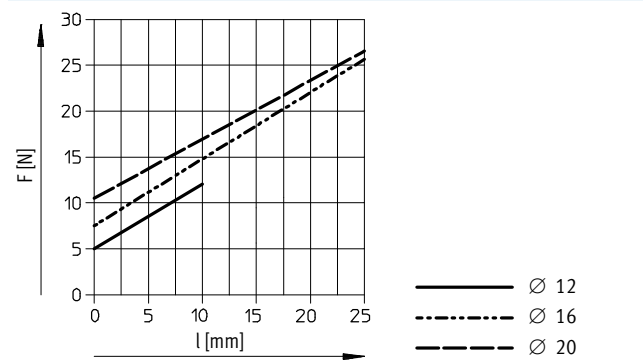
Ø 12 ... 20
