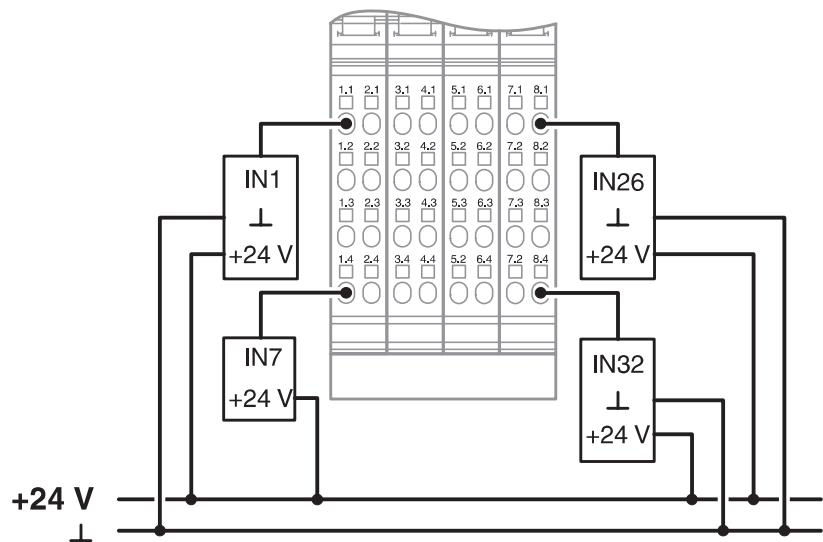
接线图
