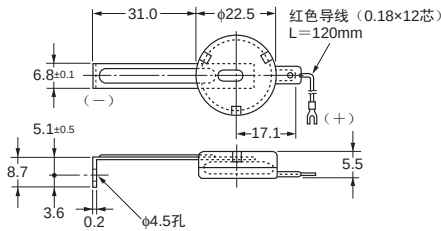
硬盖 *1 Y92A-48B
