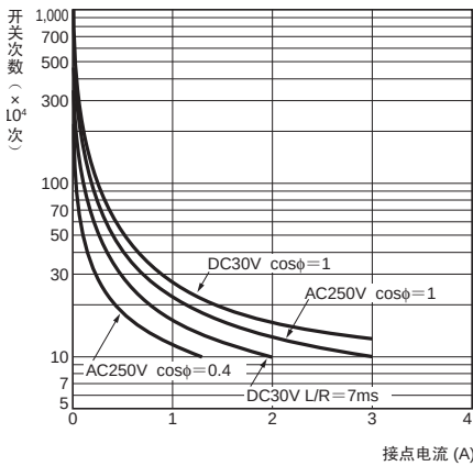
● 电气寿命曲线（参考值）
