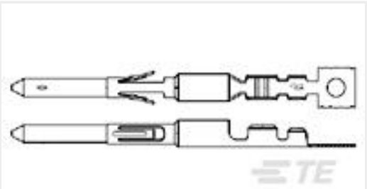
TE Part #66728-5 CIRC DIN PIN CONTACT,LP
