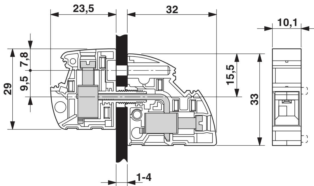
尺寸图
