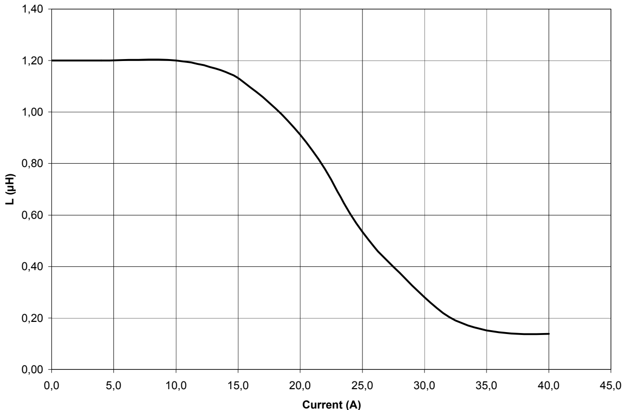
Induktivität vs Strom (typ.) / Inductance vs Current (typ.)
