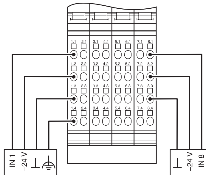
接线图
