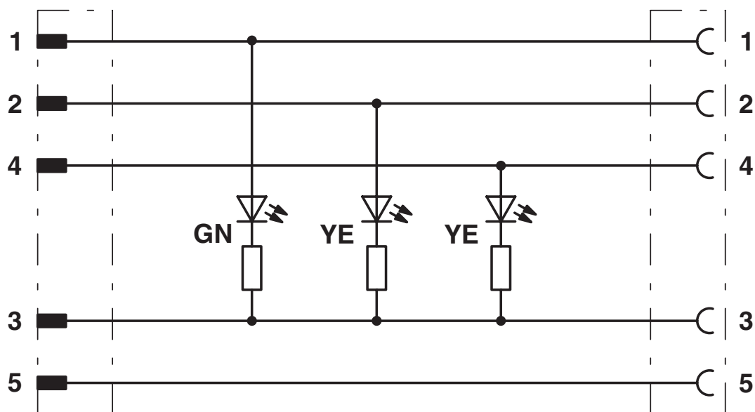
Schaltplan
