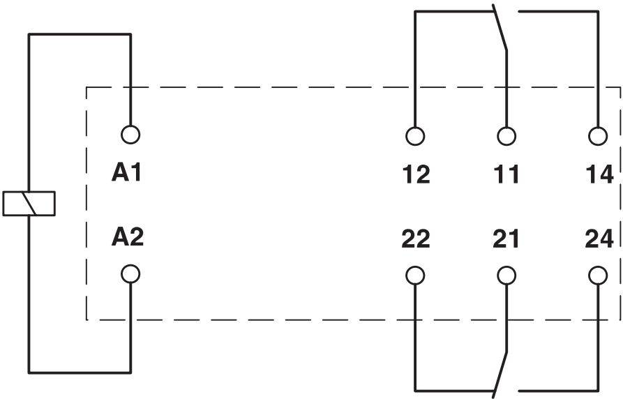
电路图
